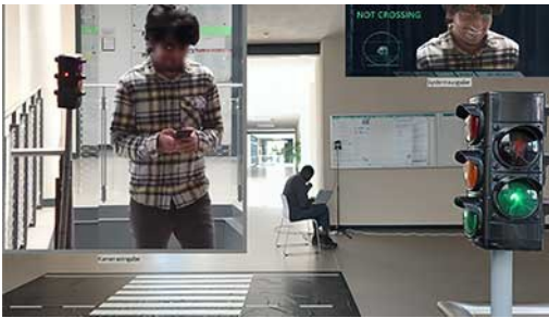
Das System zur Fußgängerabsichtsschätzung für Advanced Driver-Assistance Systems (ADAS) analysiert die Gesichtsausdrücke der Fußgänger, um ihre zukünftigen Absichten abzuschätzen.
